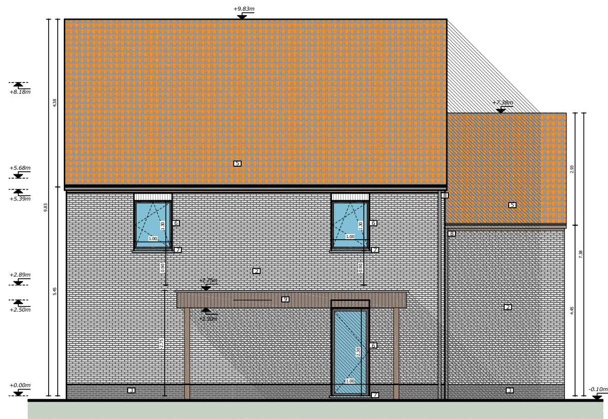
Zijgevel rechts
