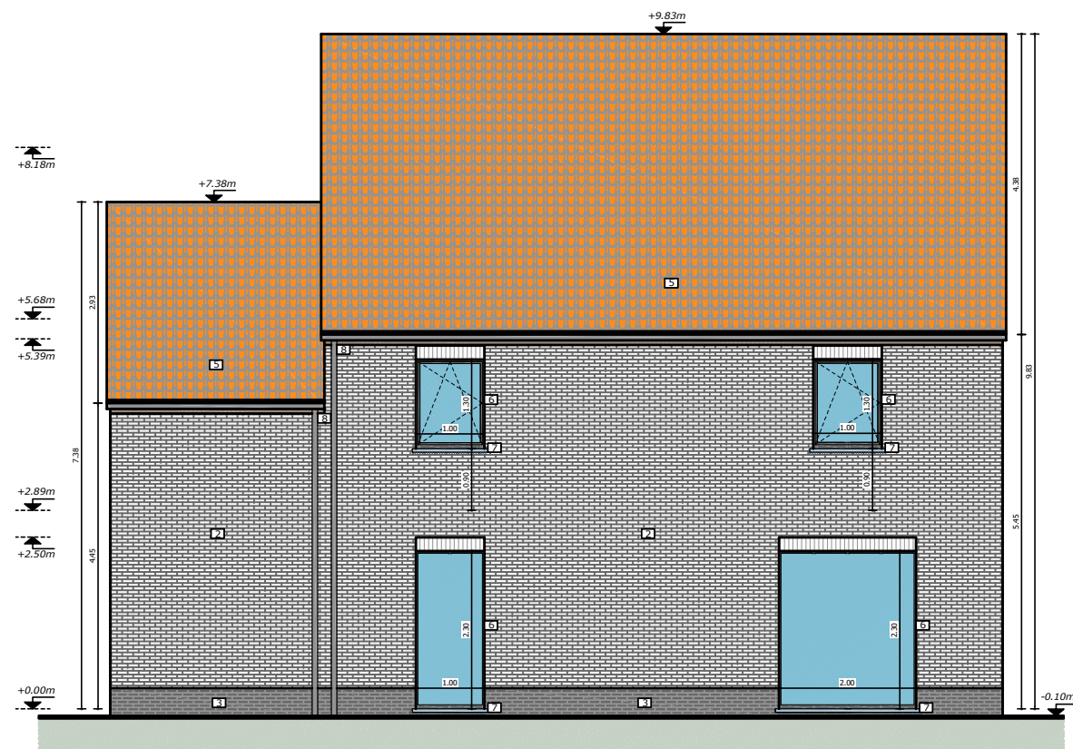
Zijgevel rechts
