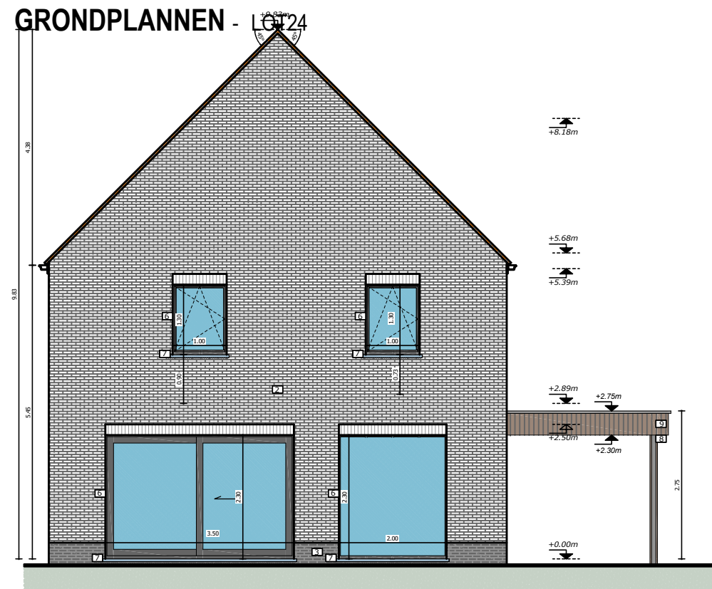
Achtergevel
